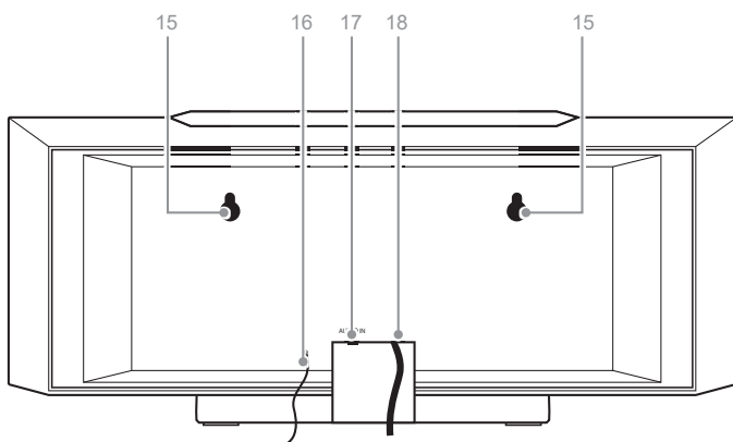
Vista posterior
