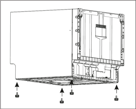
Schritt 5b: Installation der Stellschrauben
